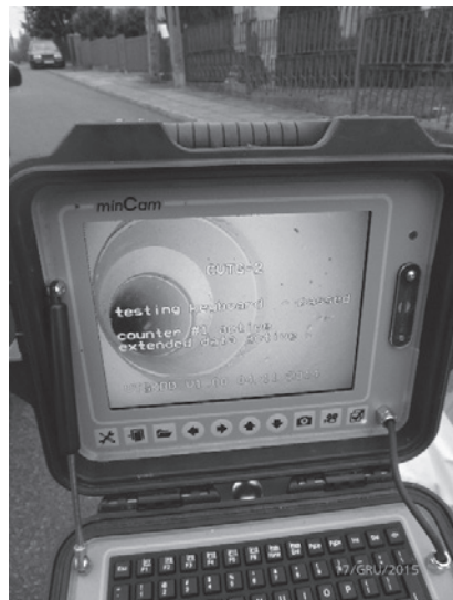
Kamera inspekcyjna umożliwia precyzyjną ocenę przebiegu i stanu kontrolowanego przewodu kanalizacyjnego.
